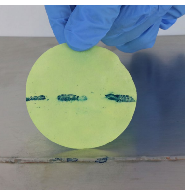
Eine Schweißnaht aus rostfreiem Stahl, die nicht ausreichend passiviert ist
